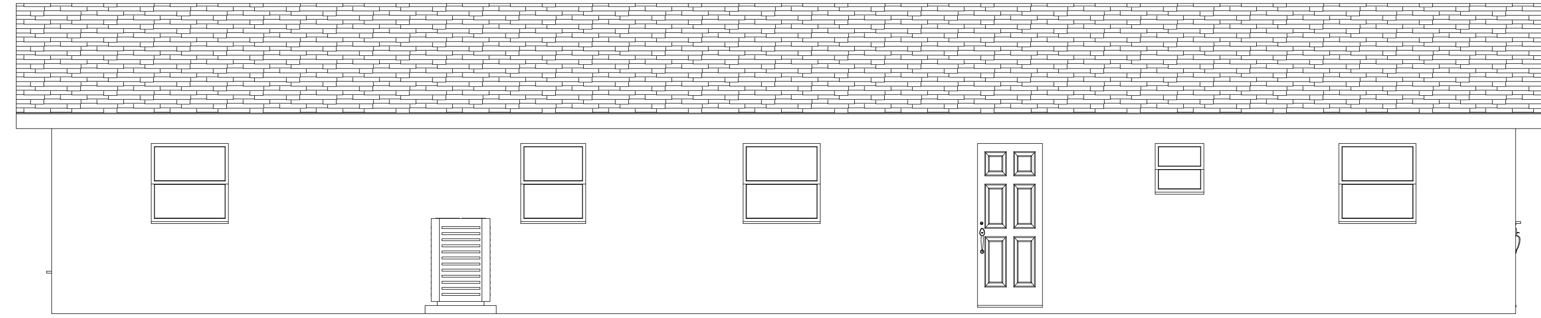
LEFT ELEVATION SCALE: 1/4" = 1'-0"
